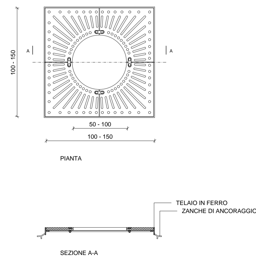
PARTICOLARE DELLA GRIGLIA PER ALBERI QUADRATA
