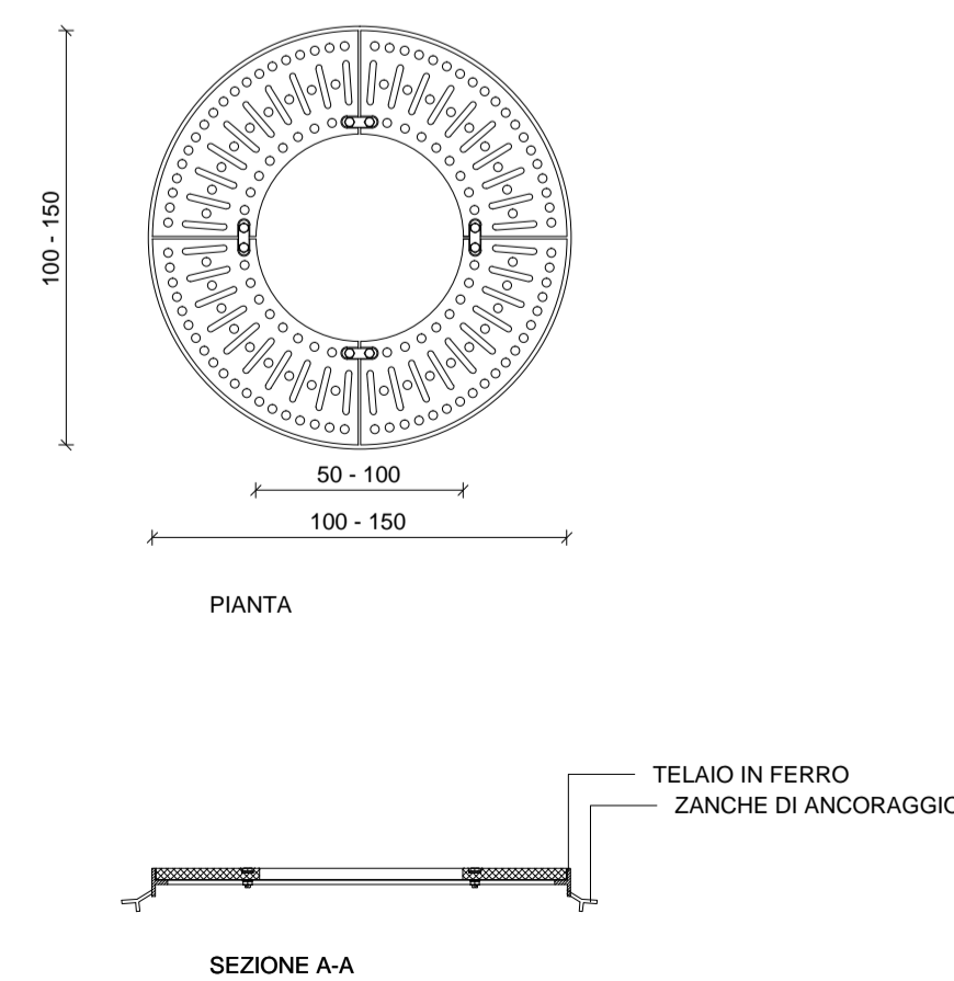
PARTICOLARE DELLA GRIGLIA PER ALBERI ROTONDA
