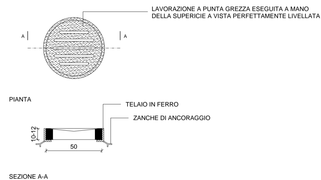
PARTICOLARE DELLA CADITOIA CIRCOLARE IN PIETRA CALCAREA
