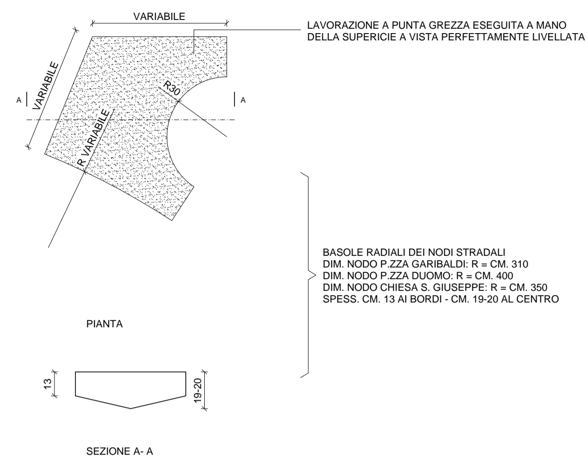
PARTICOLARE DELLE BASOLE RADIALI DEI NODI STRADALI
