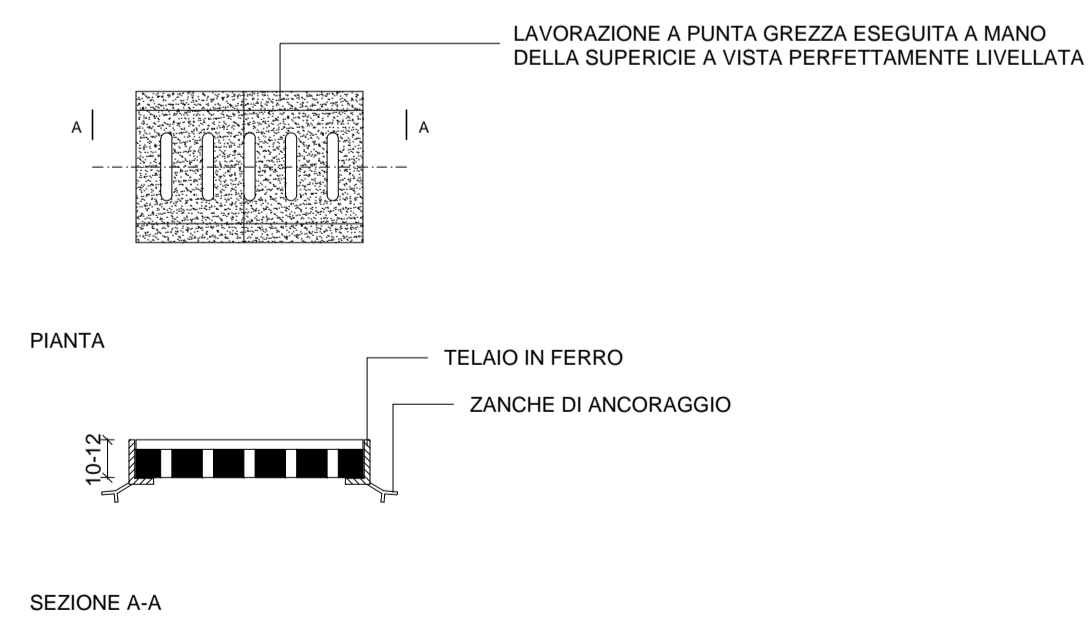
PARTICOLARE DELLA CADITOIA RETTANGOLARE IN PIETRA CALCAREA
