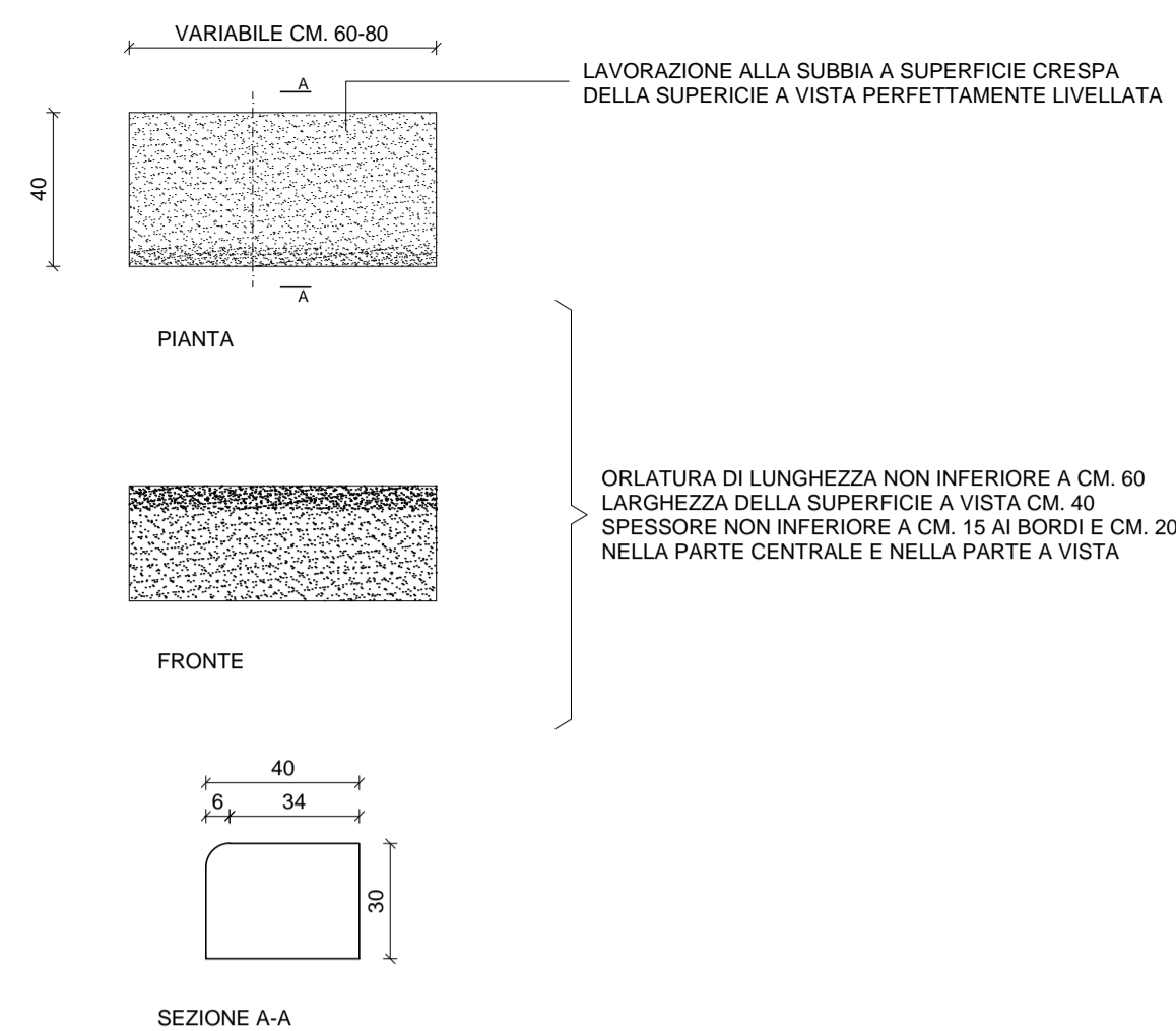
PARTICOLARE DELL'ORLATURA CON SEZIONE RETTA
