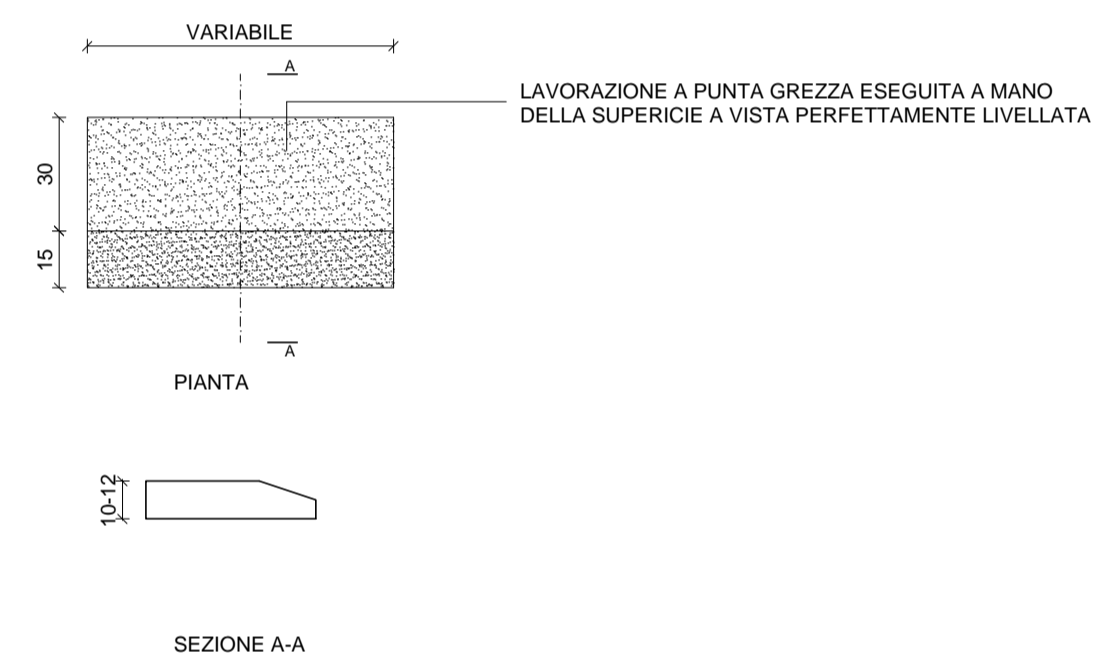
PARTICOLARE DELLE BASOLE PER PERIMETRAZIONE AIUOLE
