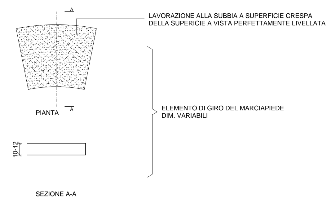
PARTICOLARE DELL'ELEMENTO DI GIRO DELLE BASOLE DEL MARCIAPIEDE
