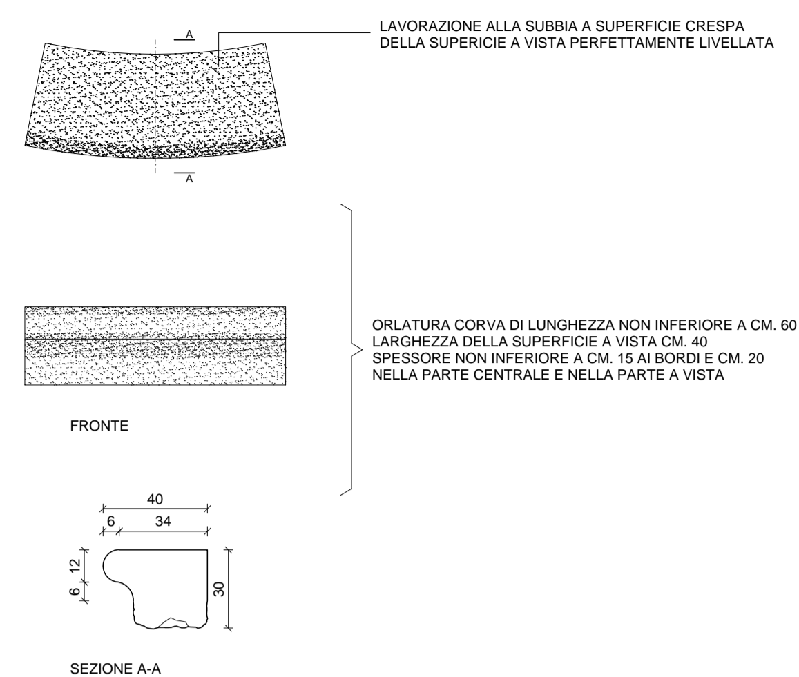
PARTICOLARE DELL'ELEMENTO DI GIRO DELL'ORLATURA CON SEZIONE A GOLA ROVESCIA
