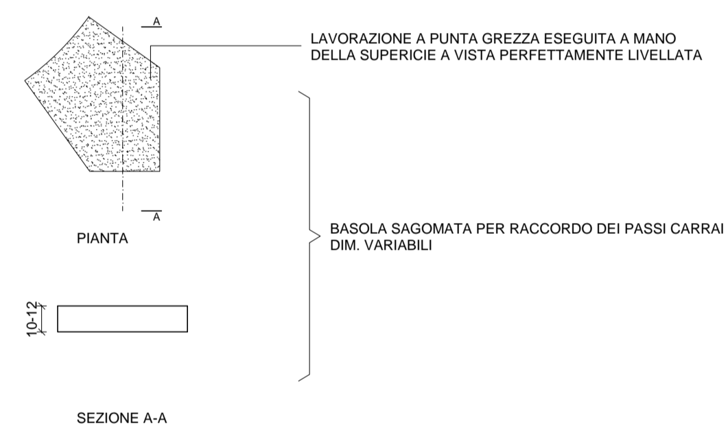
PARTICOLARE DELLE BASOLE RADIALI E SAGOMATE DI RACCORDO CON LA QUOTA STRADALE DEI PASSI CARRAI
